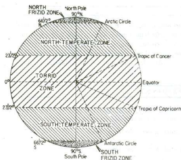
Fig. 13.1 Thermal Zone
